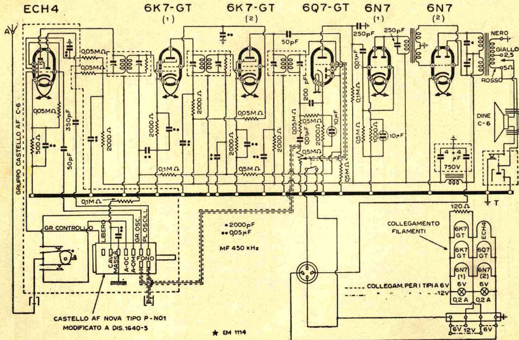
Lo schema elettrico del mod. Cyclone Six
